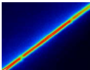
Wärmeverteilung nach ca. 30 min Betriebseinsatz der Sockelheizung.
